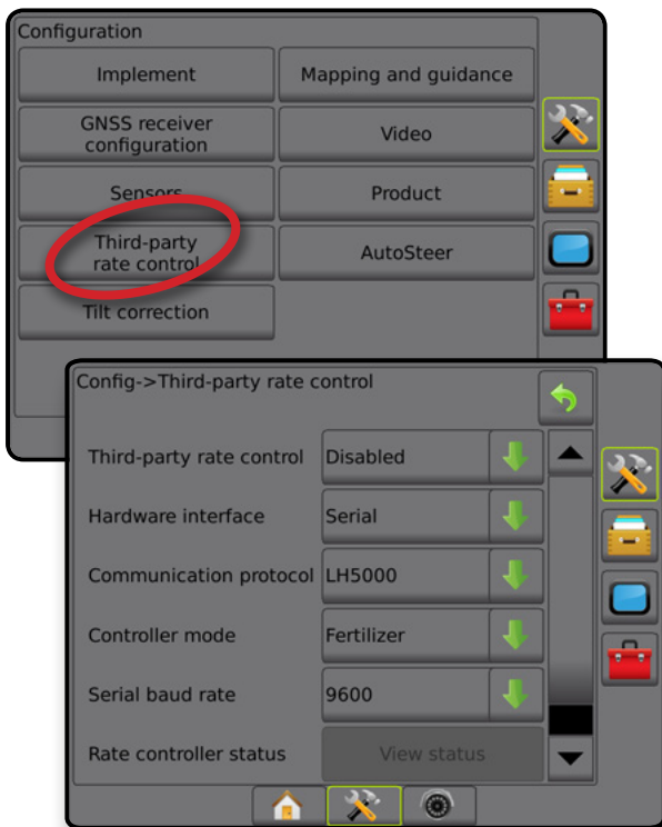
8-2 ábra: Külső cégtől származó szórás szabályozó
