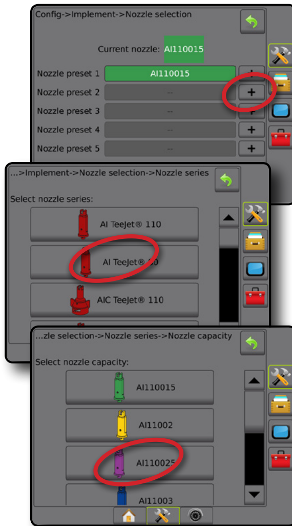
6-33 ábra: A fúvókák méretei és a hozzárendelt színek
