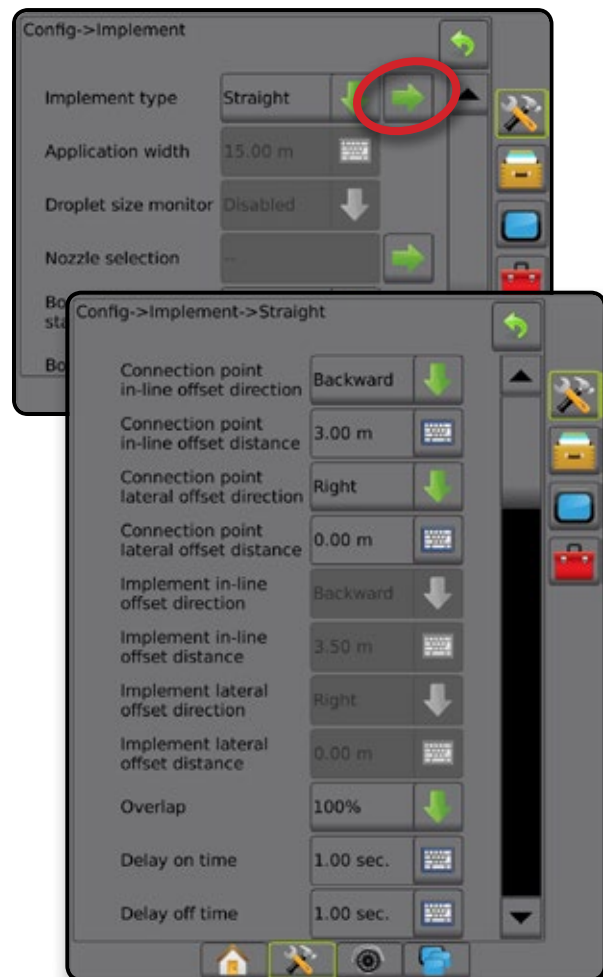
27 ábra: Egyenes szerelék típusú ISOBUS permetezőgéppel
