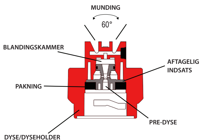
TTI60 TVÆRSNIT
