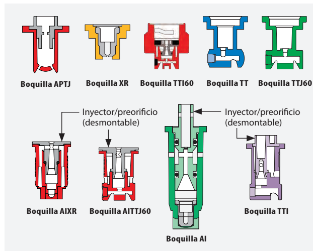
Figura 4. Vista transversal de las puntas de aspersión APTJ, XR, TT, TTJ60, AIXR, AITTJ60, AI, TTI60 y TTI.
