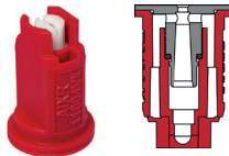
AIXR Air induction flat fan
