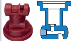
TT Turbo flat fan
